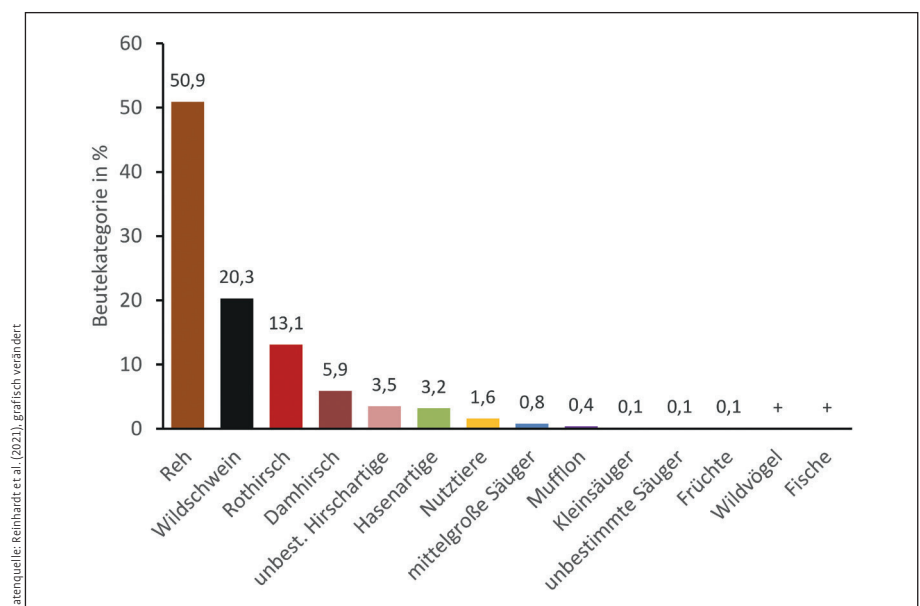
Abb. 3: Biomasseanteile der Beutekategorien/-arten in der Nahrungszusammensetzung der Wölfe in Deutschland im Zeitraum 05/2001 bis 04/2019; Kotproben: n = 8.781; „+“ \hat{=} < 0,05 %; „mittelgroße Säugertiere“ umfassen zum Beispiel Nutria ( Myocastor coypus ) und Biber ( Castor fiber ).
